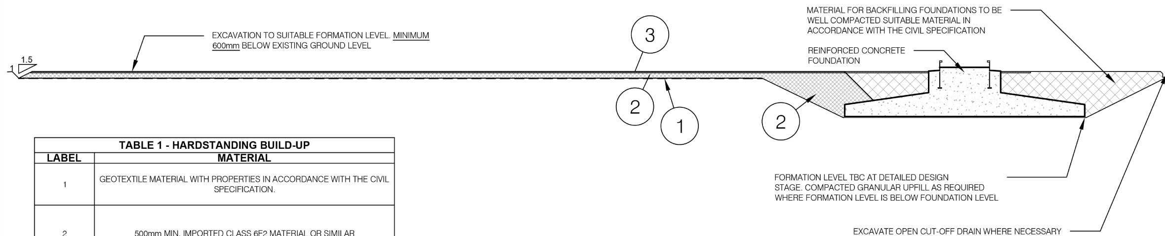
SECTION A-A
